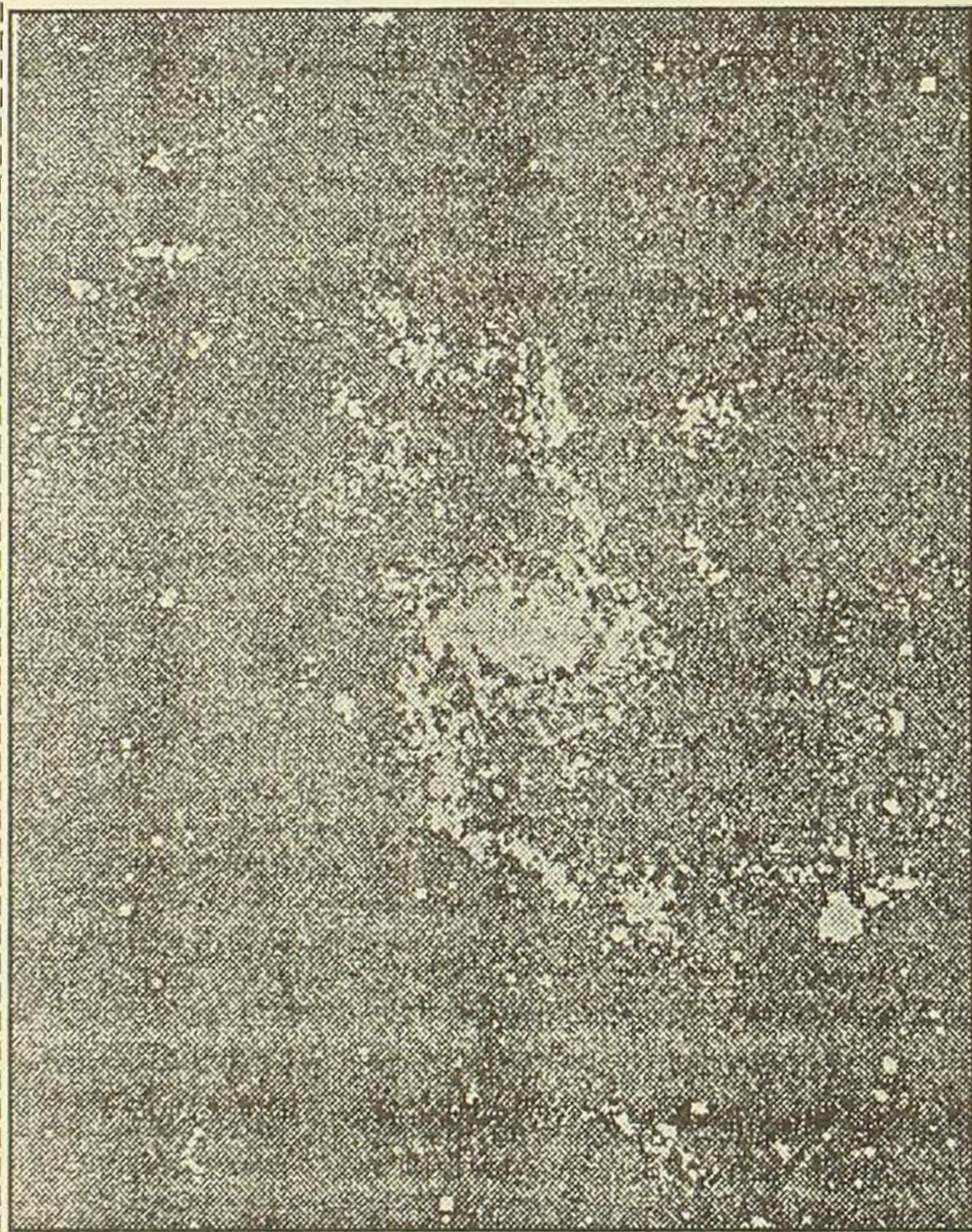
Maglina M 33 ili NGC 598 u Troughu
